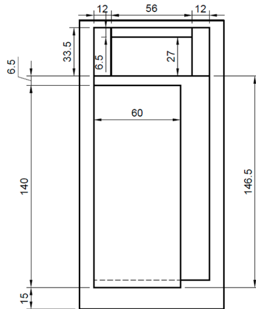
ВИД СВЕРХУ
