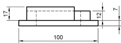
ВИД СПЕРЕДИ
