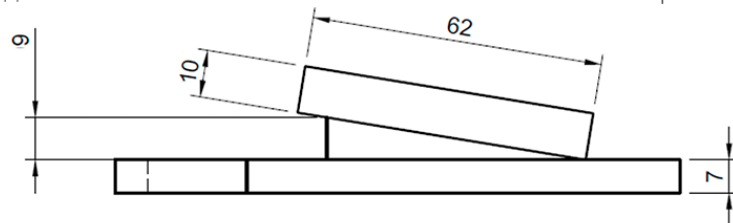
ВИД СЛЕВА
