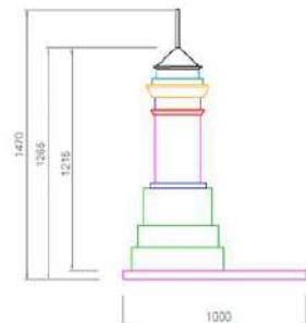
ВИД СЛЕВА
