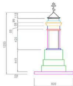
ВИД СЛЕВА
