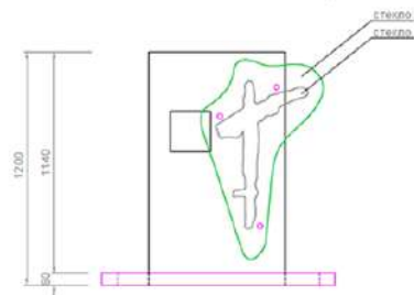
ВИД СПЕРЕДИ
